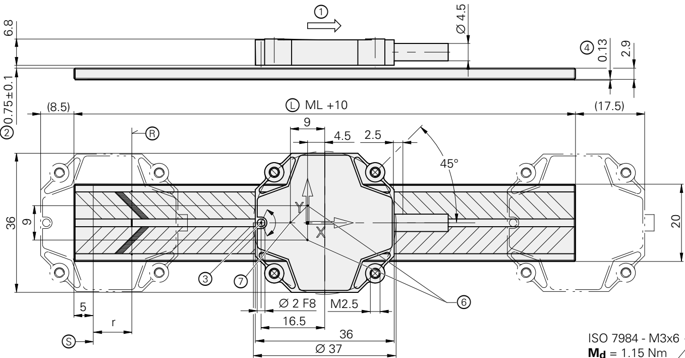
取付けに必要な寸法
