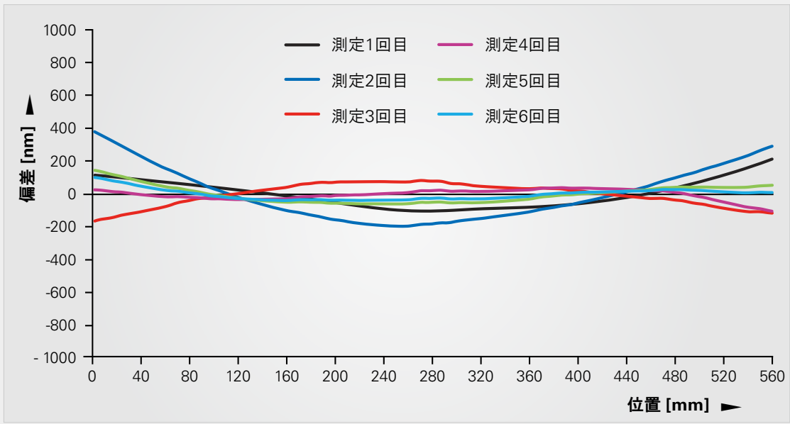
測定長に対する真直度の偏差
